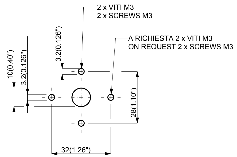
DIMA FORATURA PANNELLO DRILLING TEMPLATE
