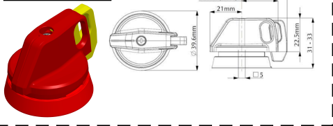
Knob
