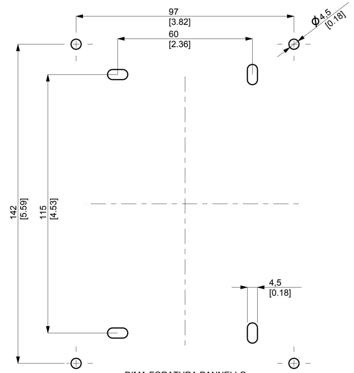
DIMA FORATURA PANNELLO DRILLING TEMPLATE
