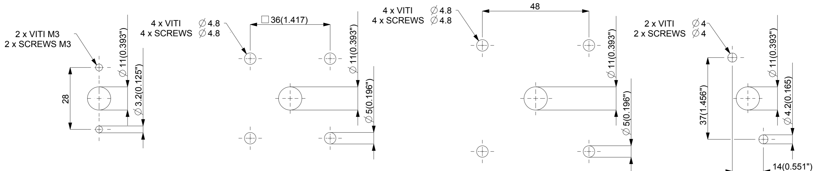
DIME FORATURA PANNELLO DRILLING TEMPLATE
