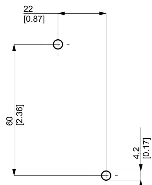
DIMA FORATURA PANNELLO DRILLING TEMPLATE
