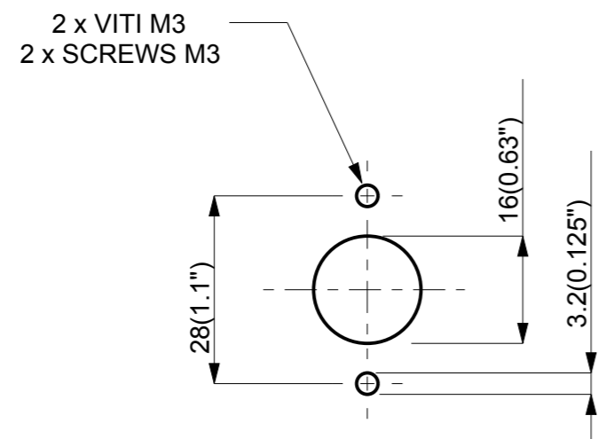
DIMA FORATURA PANNELLO DRILLING TEMPLATE
