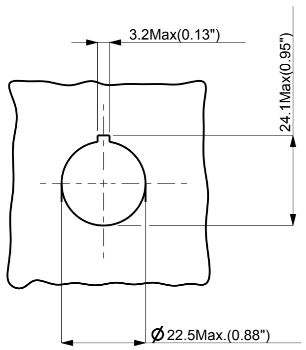
DIMA FORATURA PANNELLO DRILLING TEMPLATE
