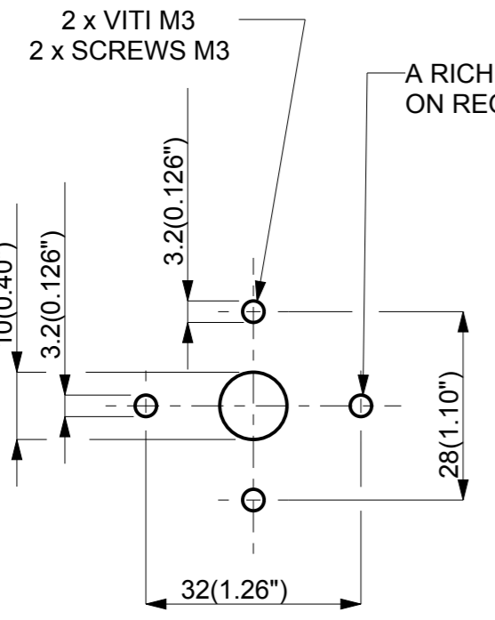
DIMA FORATURA PANNELLO DRILLING TEMPLATE
