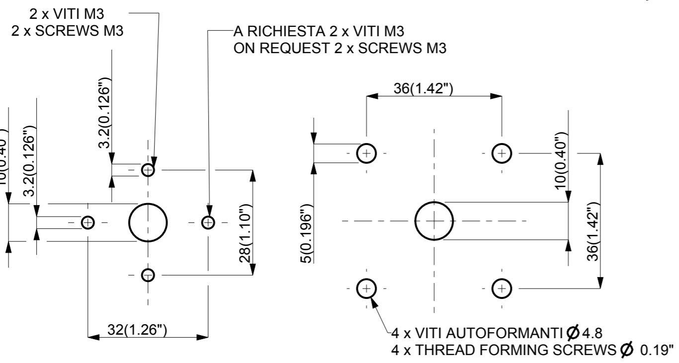
DIMA FORATURA PANNELLO DRILLING TEMPLATE
