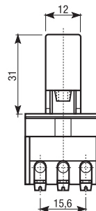
VG882500 LLA439A0 Interruttore tripolare a leva arancio instabile, senza fori fissaggio
