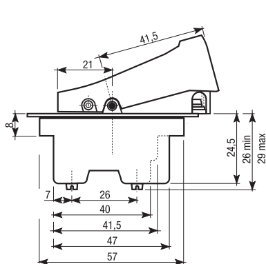
VG882500 LLA439A0 Interruttore tripolare a leva arancio instabile, senza fori fissaggio
